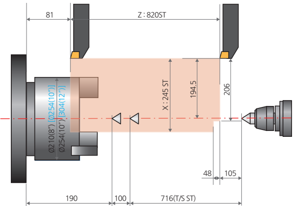
O.D Tool
