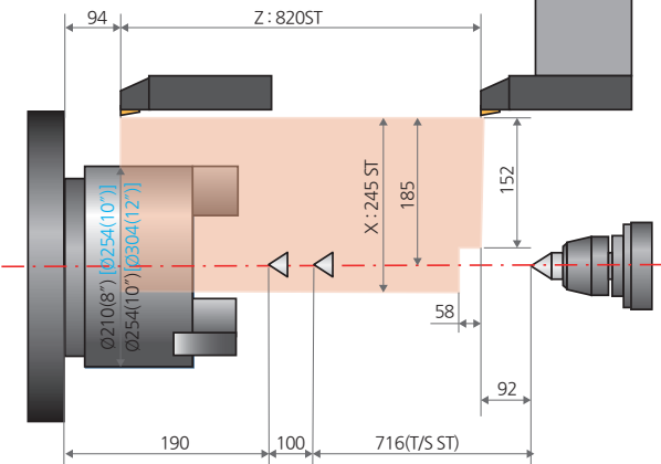
FACE Tool
